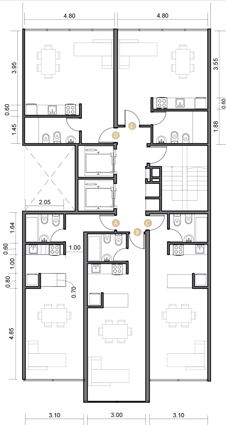
PLANTA TIPO
